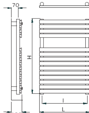
H080 - 14 TUBOS
